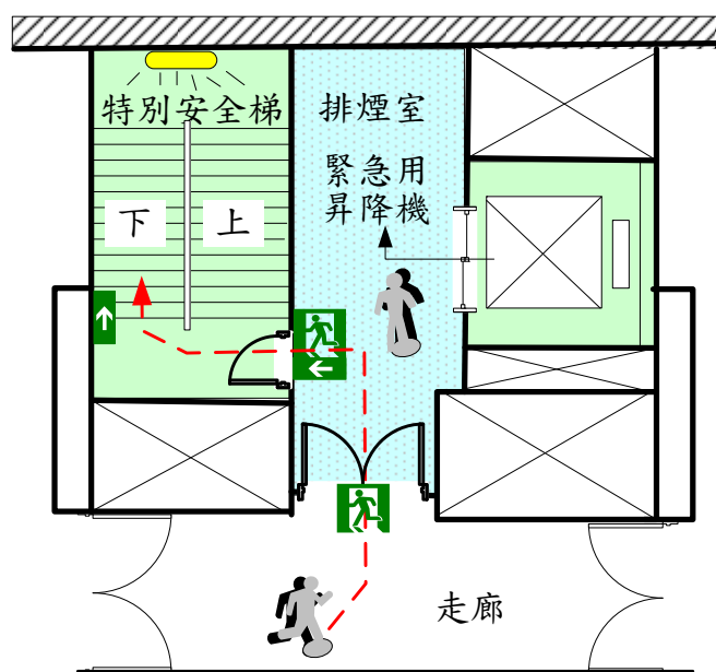
圖 2-13 排煙室
