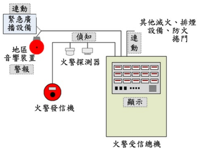
圖 2-28 火警自動警報設備架構圖
