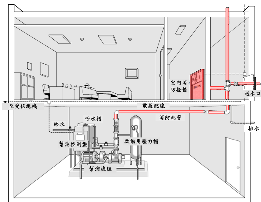
圖 2-19 室內消防栓系統圖 (資料來源：同註 1)
