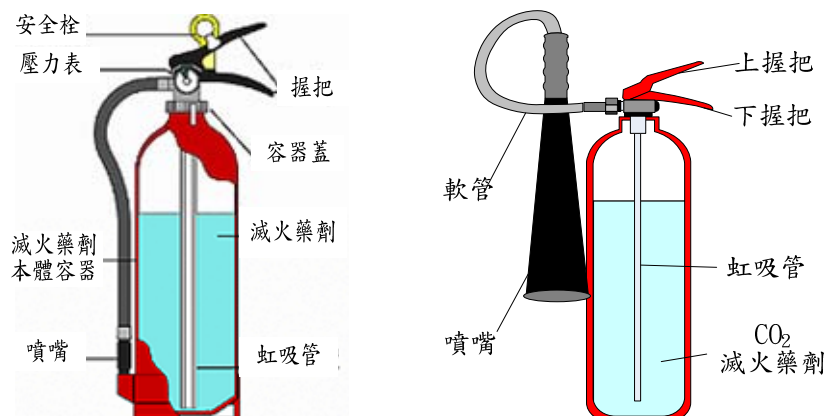
圖 2-16 蓄壓式滅火器構造 （資料來源：同註 1）
