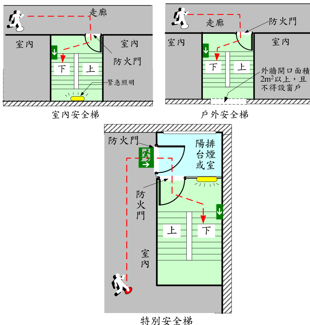
圖 2-11 安全梯示意圖
