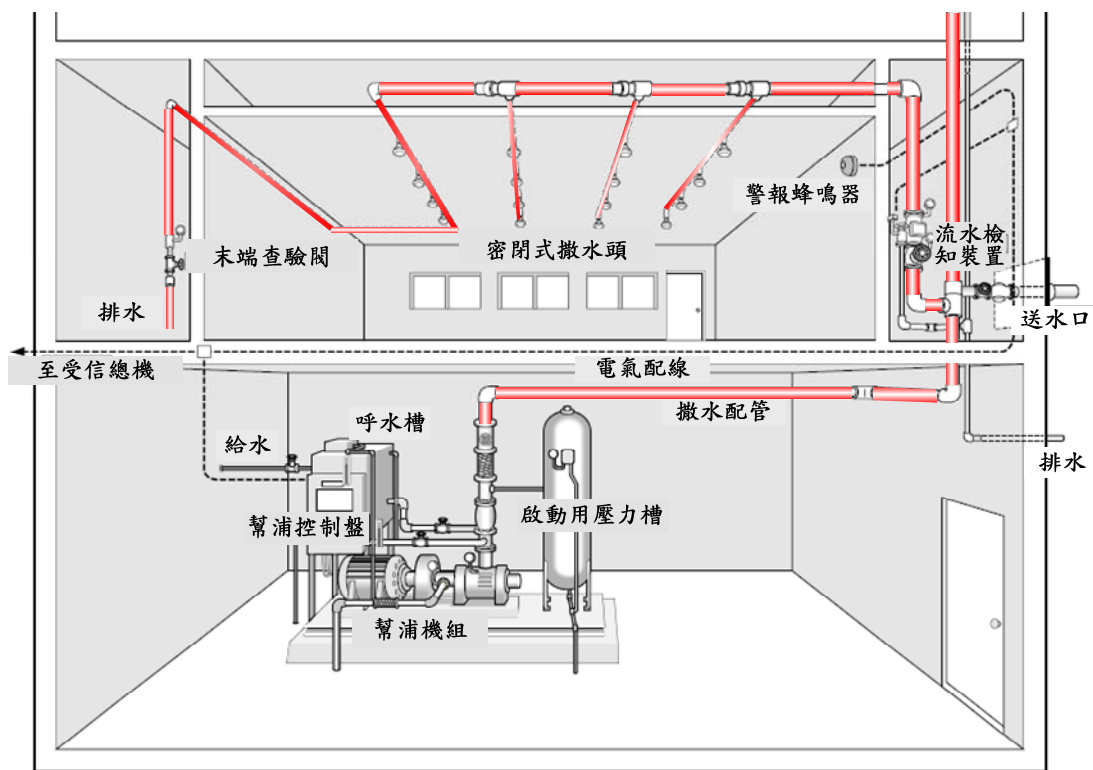
圖 2-23 自動撒水設備系統圖 (資料來源：同註 1)
