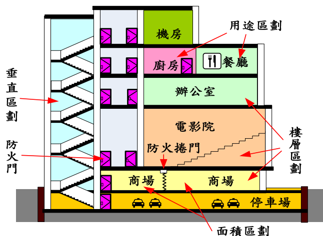
圖 2-3 防火區劃種類示意圖
