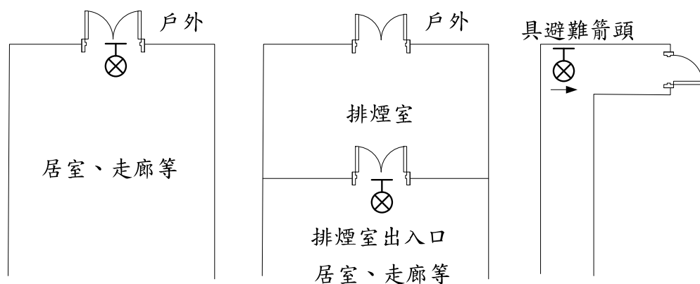
圖 2-6 通往戶外逃生出入口例
