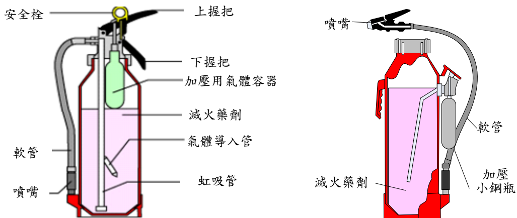
圖 2-17 加壓滅火器構造
