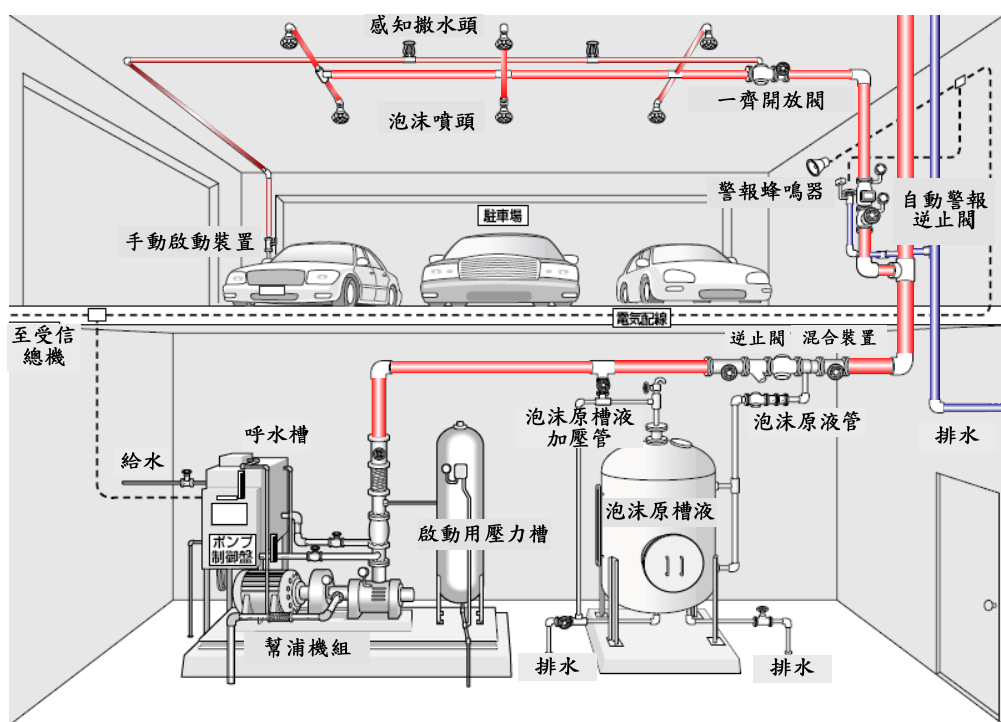
圖 2-26 泡沫滅火設備系統圖（資料來源：同註 1）
