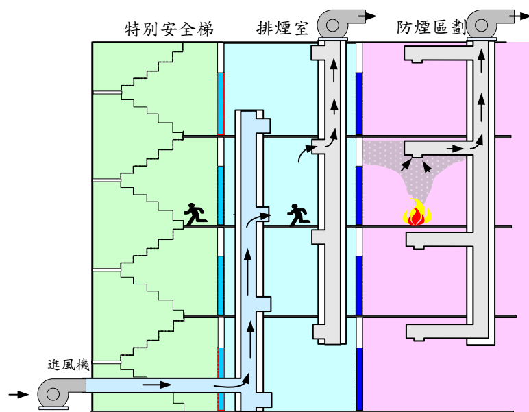
圖 2-35 排煙設備示意圖
