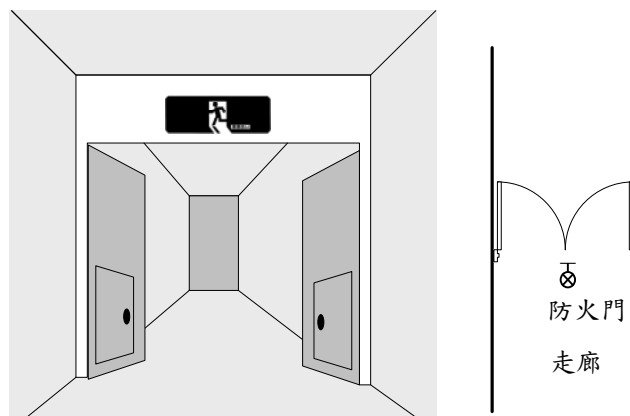
圖 2-9 通往另一防火區劃之防火門例
